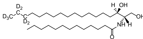
13:0-18:0(d7) dHCer
