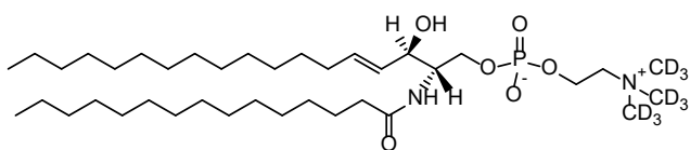
15:0-18:0 SM (d9)
