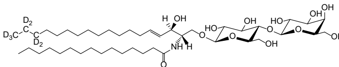
15:0-18:1(d7) LacCer
